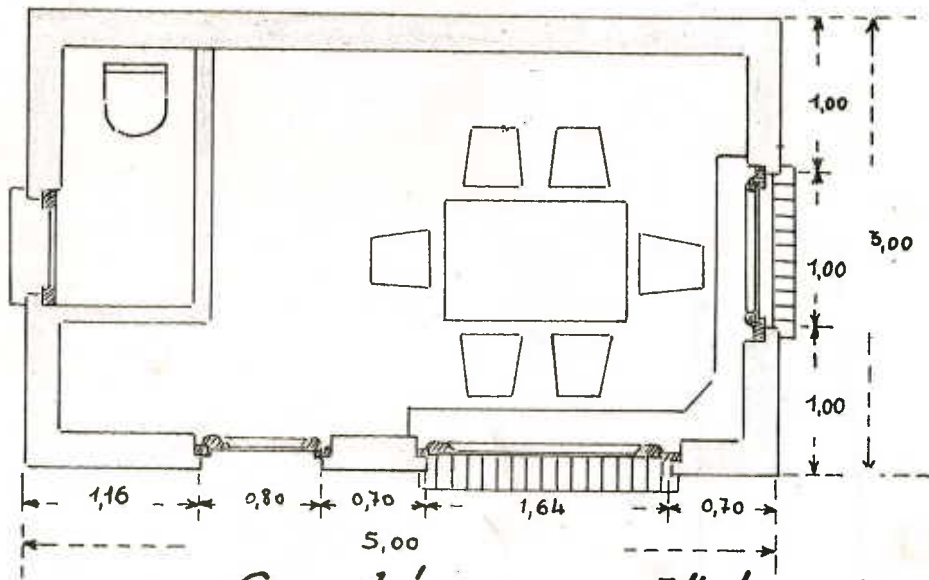
Grundriss
