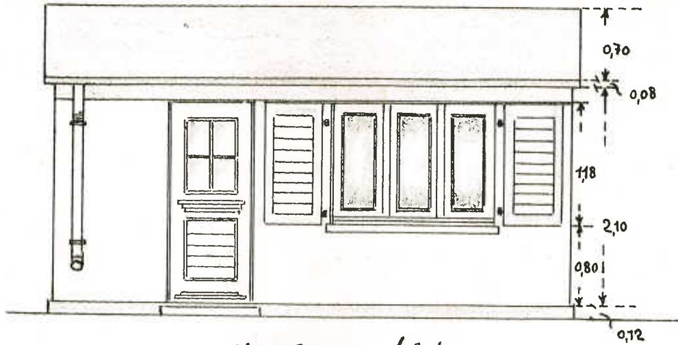
Vorderansicht
